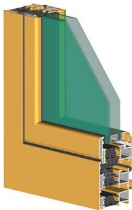
Sistema de batente com RPT - 75 mm
